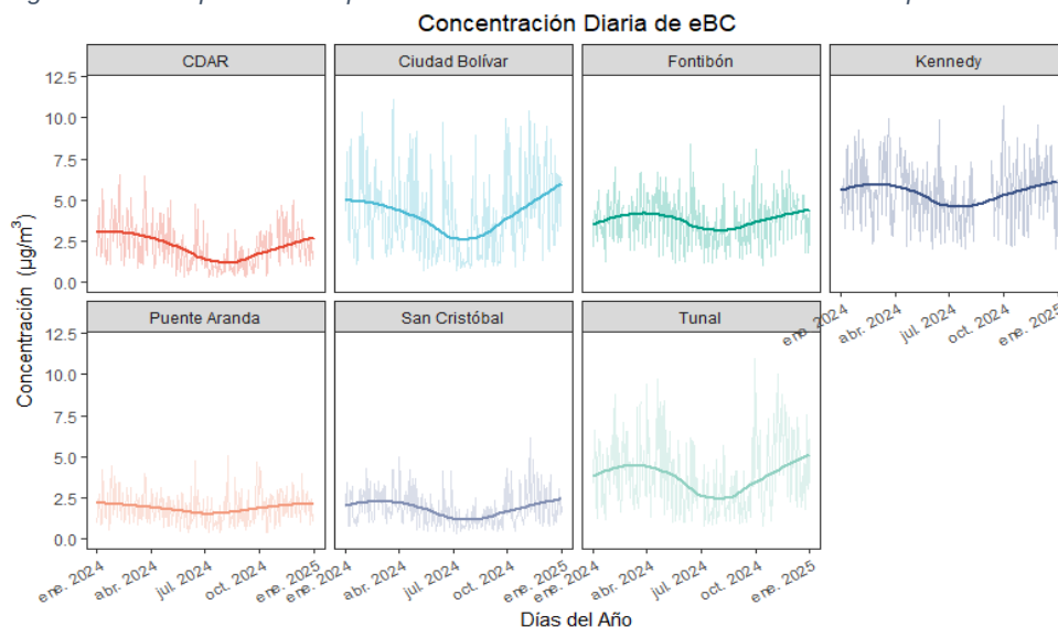
Figura 8-2. Comportamiento promedio diario de las concentraciones de eBC para el 2024.
