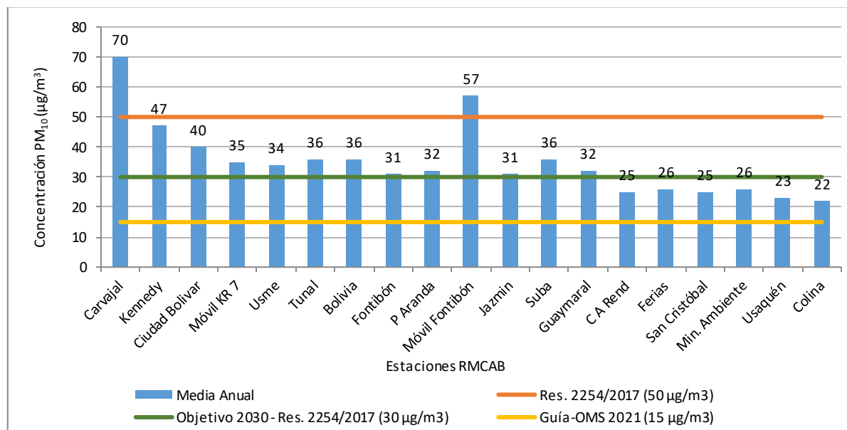
Figura 12-12 Concentración promedio y excedencia a la normativa Guía-OMS y Resolución 2254 de 2017 de PM 10 , para estaciones de la RMCAB, 2024
