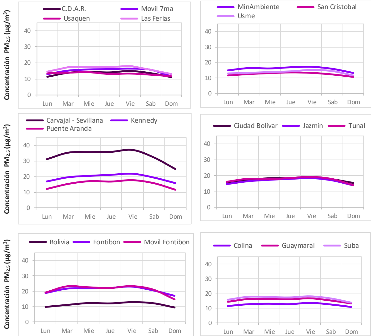
Figura 7-10 Comportamiento diario de las concentraciones de PM_{2.5} – Año 2024
