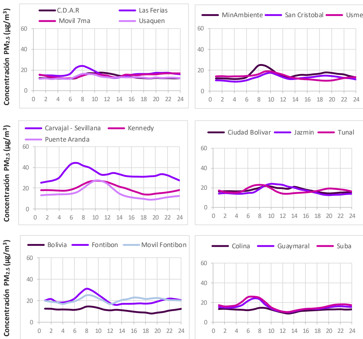
Figura 7-11 Comportamiento horario de las concentraciones de PM_{2.5} – Año 2024
