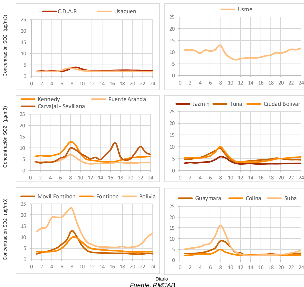
Figura 7-29 Comportamiento horario de las concentraciones de SO 2 – Año 2024
